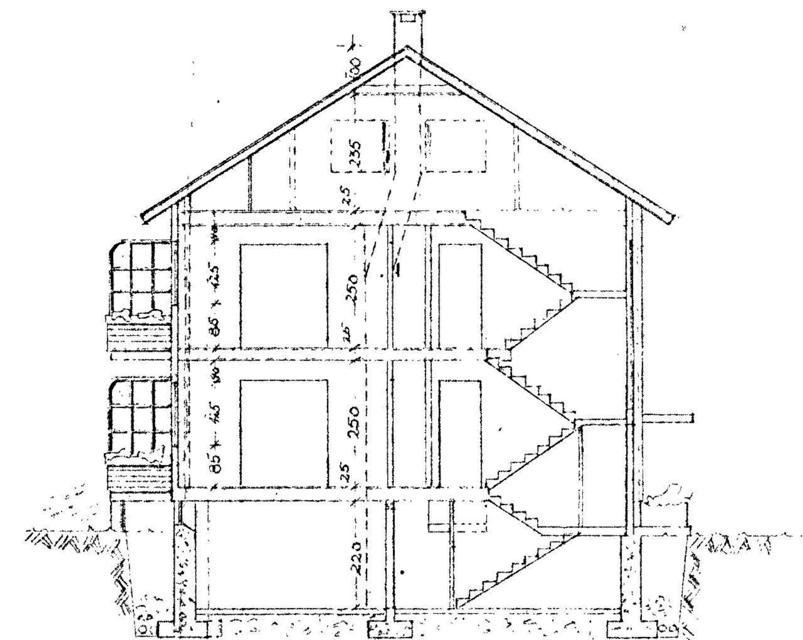
Snitt 1-2
